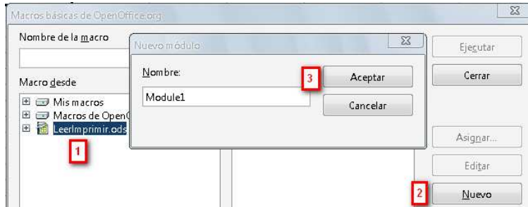
Figura 1.4 Crear Módulo
