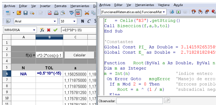
Figura 1.2 OOo Calc
